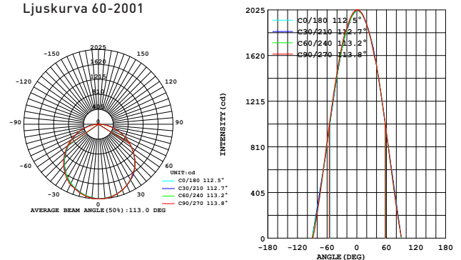
Ljuskurva 60-2001
