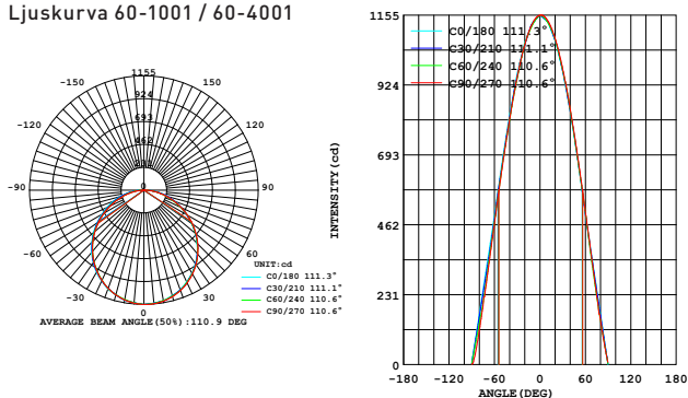
Ljuskurva 60-1001 / 60-4001
